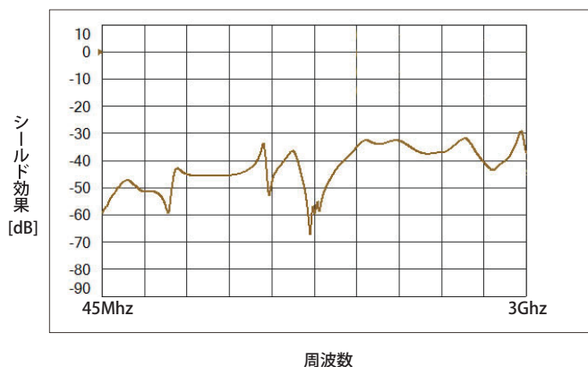
●周波数とシールド効果
