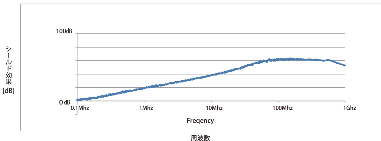
●周波数とシールド効果（磁界）
