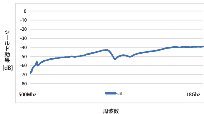
●周波数とシールド効果
